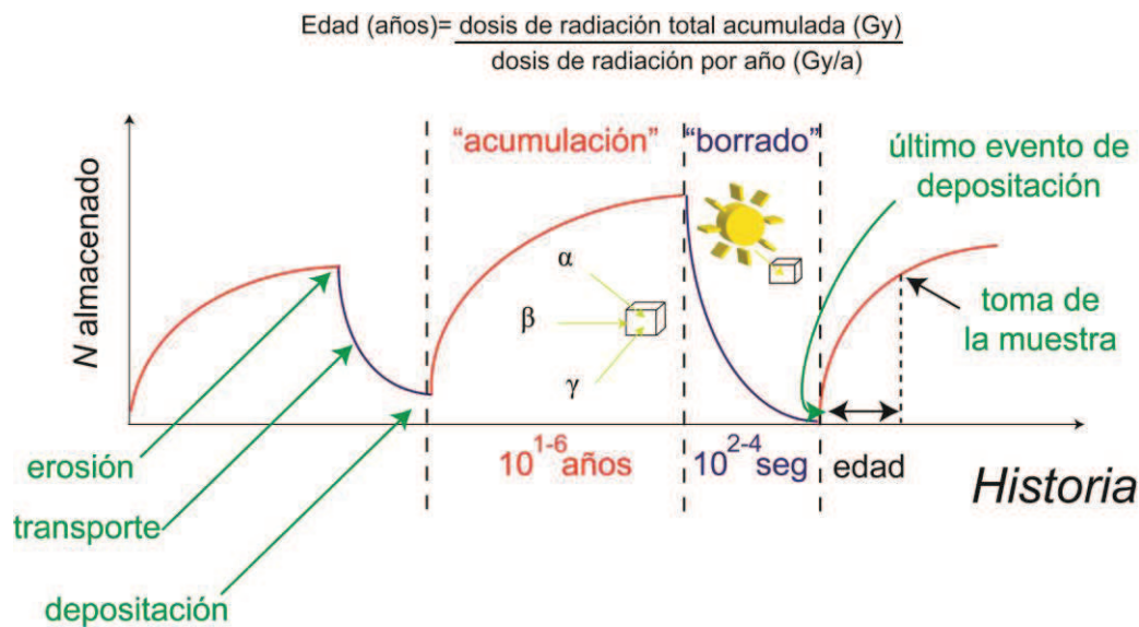
Figura 1.16. Esquema que muestra las etapas de acumulación de radiación ionizante y la liberación de las cargas mediante luminiscencia. Las líneas rojas indican incremento de radiación ionizante ( N ). Las líneas azules representan el “reseteo” del sistema, que implica la liberación de la señal acumulada debido a procesos de transporte y erosión. El material, al enterrarse nuevamente, comienza a acumular nuevamente la radiación ( N ). Se indica además la fórmula utilizada para el cálculo de la edad (Imagen del sitio web USGS, autorizada por el Dr. K. Lepper, North Dakota State University)
