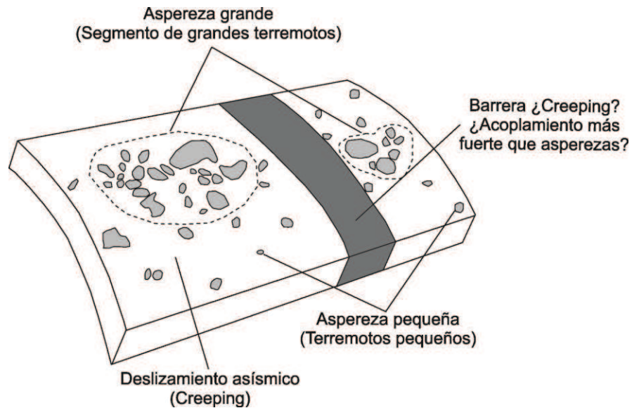
Figura 1.6. Asperidades y barreras en una zona sismogénica interplaca. Modificado de Kaneko et al. [2010].
