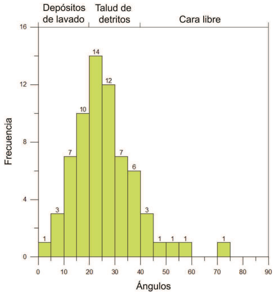
Figura 4.5. Muestra los ángulos dominantes a lo largo de perfiles hechos en el escarpe principal de la Falla Salar del Carmen. Los ángulos menores a 20° corresponden a los depósitos de lavado, aquéllos entre 20° y 40° al talud de detritos, y las inclinaciones sobre 40° a la cara libre.
