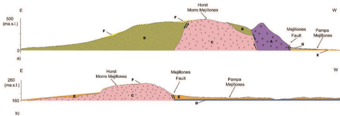
Figura 1.12. Secciones esquemáticas hacia la parte norte (a) y sur (b) del horst de Morro Mejillones y Pampa Mejillones. A= Rocas intrusivas paleozoicas; B= Rocas metamórficas paleozoicas; C= Rocas intrusivas mesozoicas; D= Lavas andesíticas de la Fm. La Negra; E= Depósitos marinos miocenos-pleistocenos en Pampa Mejillones; F= Depósitos marinos pleistocenos en Horst Morro Mejillones; G= Depósitos aluviales cuaternarios.
