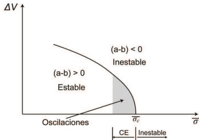
Figura 1.9. Tomada de Scholz [1998]. Gráfico que muestra los dominios estable, inestable y condicionalmente estable (CE). \Delta V es el cambio de velocidad y \sigma es el stress normal. \sigma_c es el stress normal crítico para pasar desde un régimen estable (condicionalmente) a inestable.
