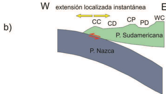
Figura 1.13. Representación esquemática de los procesos que favorecen: a) Extensión por medio de erosión por subducción y underplating ; y b) Extensión cosísmica. MS= Manto superior; CC= Cordillera de la Costa; CD= Depresión Central; CP= Precordillera; PD= Depresión preandina; WC= Cordillera Occidental. Modificada de Delouis et al., [1998].
