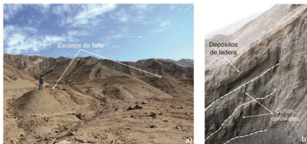
Figura 2.1. a) Escarpe de falla. b) Cuña coluvial. Ambos rasgos constituyen evidencias paleosismológicas primarias, la primera de naturaleza geomorfológica, y la segunda de tipo sedimentaria.
