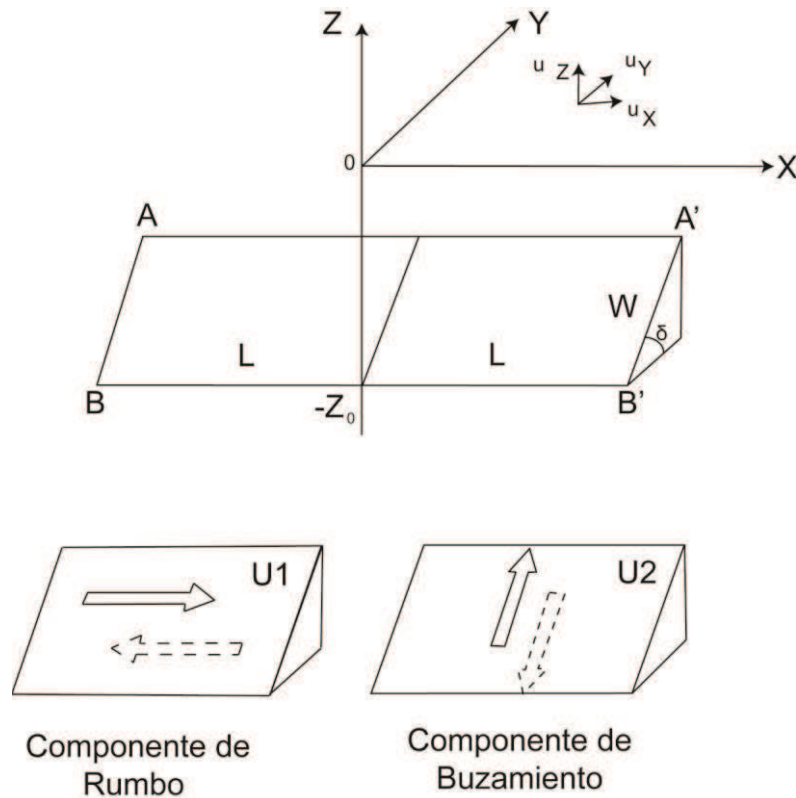
Figura 5.3. Tomada de Ruegg [1994]. Geometría del modelo de fuente rectangular en el sistema de referencia de Okada [1985].
