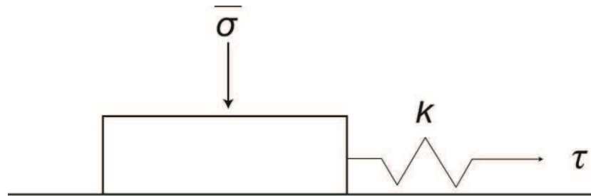
Figura 1.8. Tomada de Scholz [1998]. Ilustra el experimento simple a partir del cual se determinan los regímenes de estabilidad. \sigma es el stress normal, k la constante de elasticidad y \tau el stress de cizalle.
