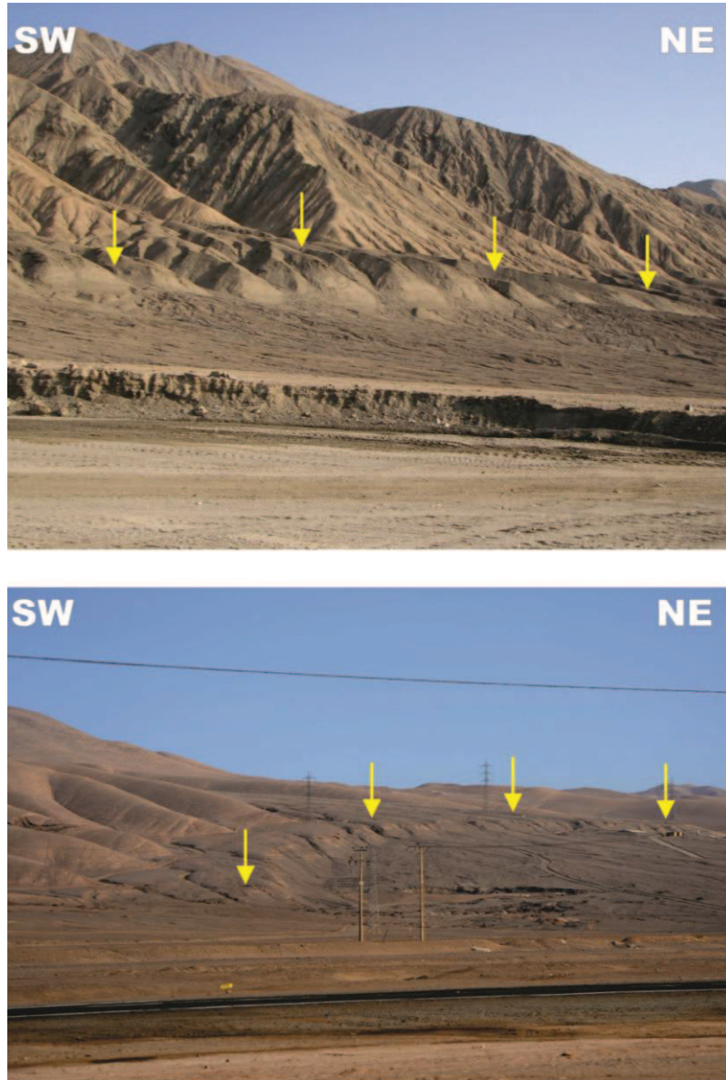
Figura 1.11. Aspecto general de las fallas Mejillones (a) y Salar del Carmen (b). Ambas estructuras afectan depósitos aluviales cuaternarios, como lo indican las flechas amarillas.
